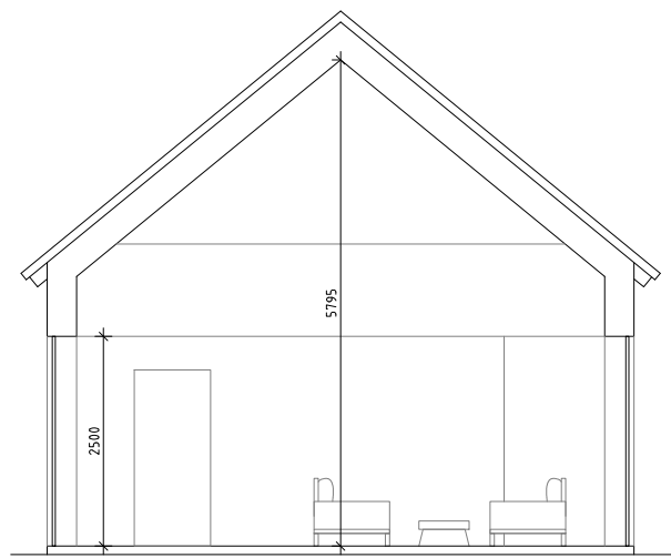
SEKTION A-A
