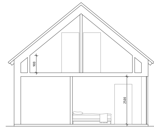
SEKTION C-C
