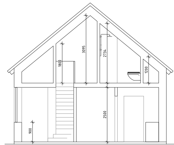
SEKTION B-B
